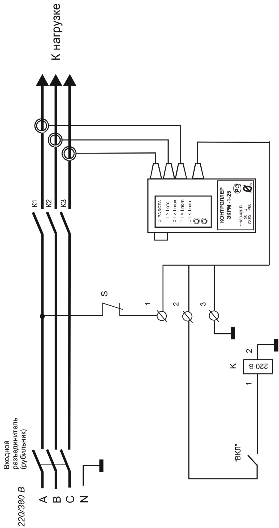
Рисунок 4 - подключение контроллера в схему управления контактора с самозапуском при восстановлении питания
