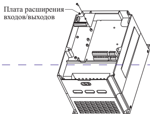
Способ установки платы расширения входов/выходов
