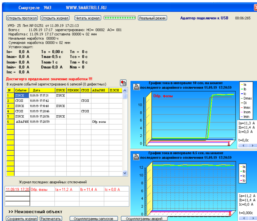
Рисунок 8 – отображение журнала аварийных отключений Смартреле УМЗ на экране ПК
