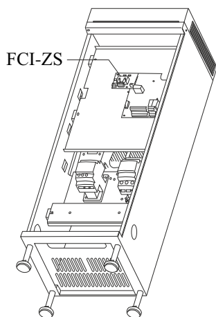
Способ установки FCI-ZS
