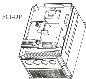
Способ установки FCI-DP
