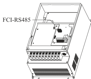
Способ установки FCI-RS485
