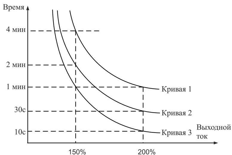
Обратнoзависимые кривые перегрузки
