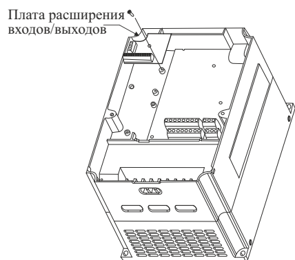
Способ установки платы расширения входов/выходов
