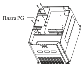
Способ установки платы расширения PG
