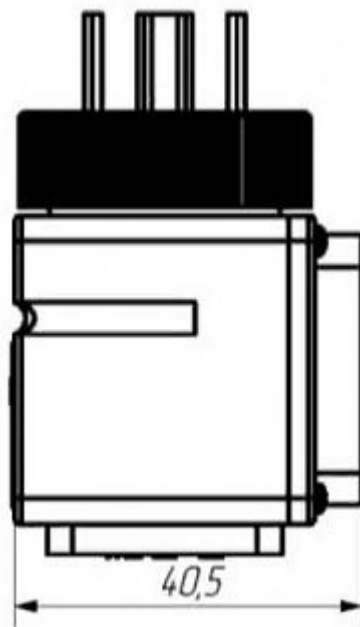
Вилка DIN 43650 A
