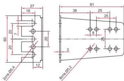
Кронштейн реле температуры
