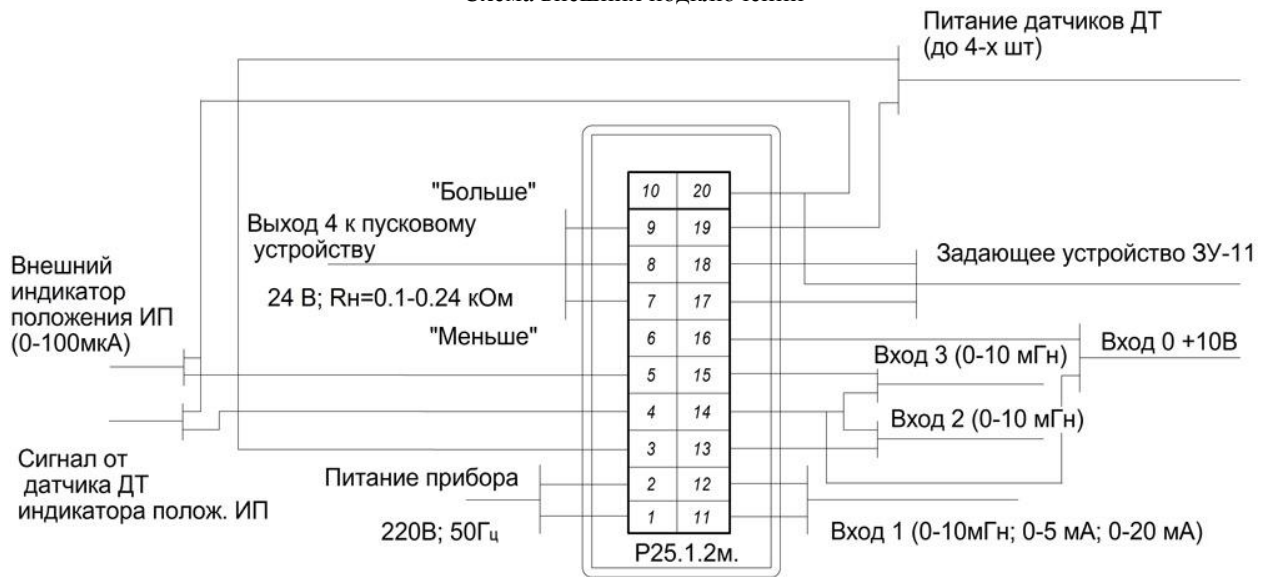
Схема подключения прибора P25.1.2м.
