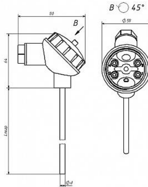
ТСП-101-M20x1,5, ТСП-К-101 –M20x1,5.
