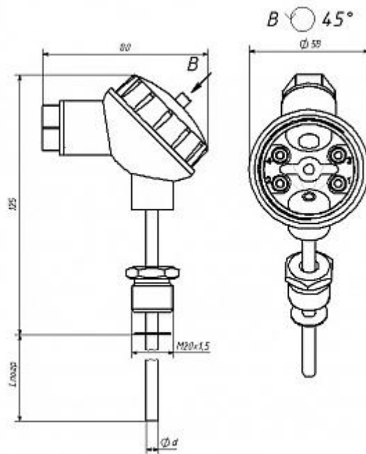
ТСП-101-M20x1,5, ТСП-К-101 –M20x1,5.
