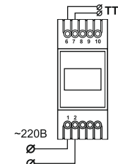
Схема подключения
