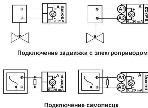
Рисунок 13 – Схемы подключения аналогового выхода
