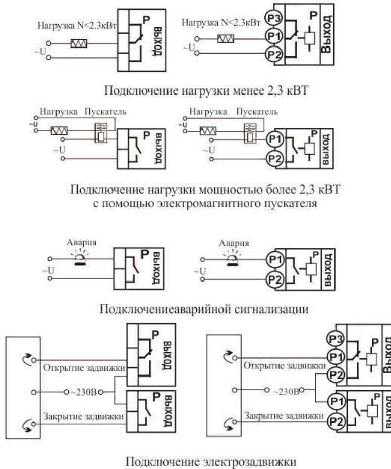
Рисунок 12 – Схемы подключения релейных выходов
