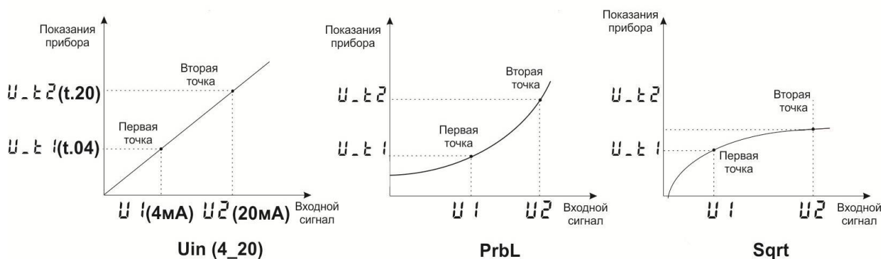
Рисунок 9 – Графики зависимости показаний прибора от входного сигнала при использовании входа типа U.in, PrbL, Sqrt и датчика 4...20
