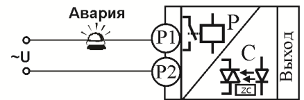
Подключение аварийной сигнализации
