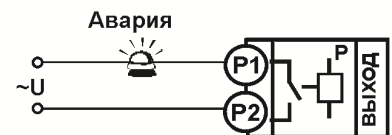
Подключение аварийной сигнализации
