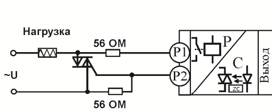
Подключение внешнего симистора
