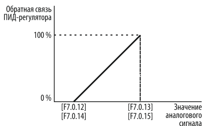
Рисунок 161 – масштабирование обратной связи ПИД-регулятора относительно аналогового сигнала.
