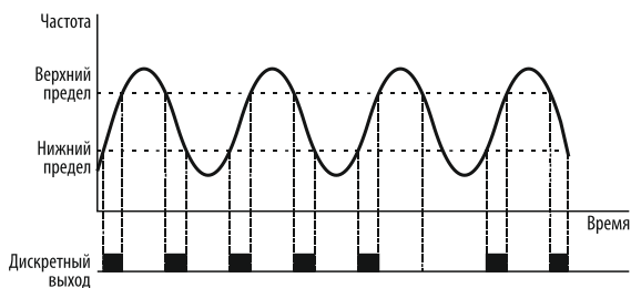
Рисунок 105 – включение дискретного выхода при нахождении параметра мониторинга между значениями верхнего и нижнего предела.
