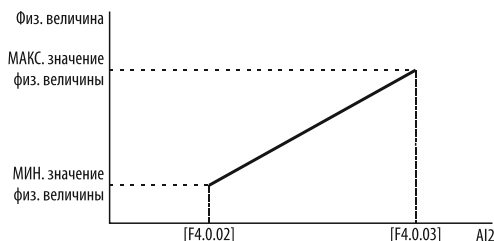
Рисунок 112 – минимальное и максимальное значение тока на аналоговом входе AI2 .
