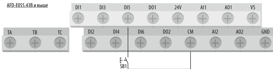
Рисунок 53 – схема подключения цепей управления при [F0.0.00] = «1» для AFD-E055.43B и выше.
