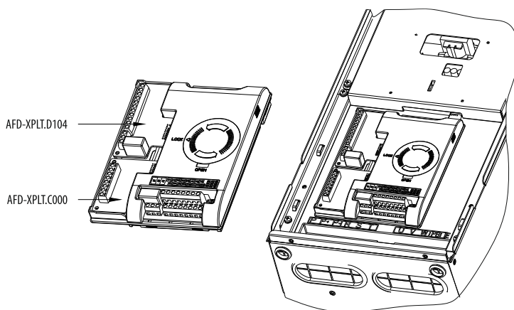
Рисунок 176 – установка карт расширения в преобразователи частоты AFD-E055.43B и выше
