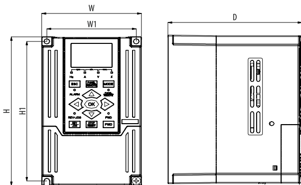
Рисунок 13 – габаритные размеры ПЧ AFD-E040.43B и ниже (тип корпуса 1, габариты 1, 2)
