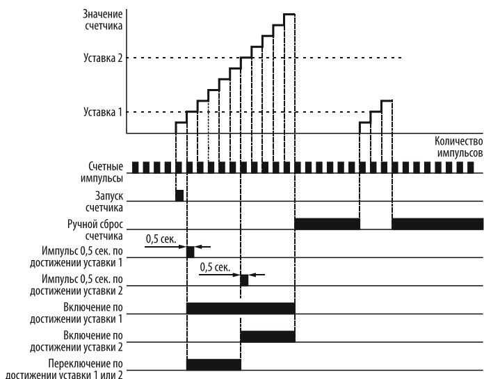
Рисунок 144 – ручной сброс текущего значения счетчика по сигналу на дискретном входе.
