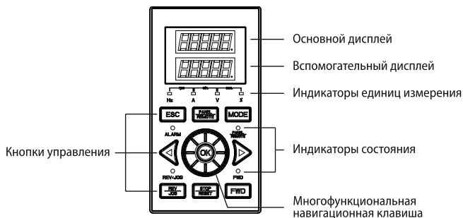
Рисунок 8 – внешний вид панели управления AFD-XPNL.22.
