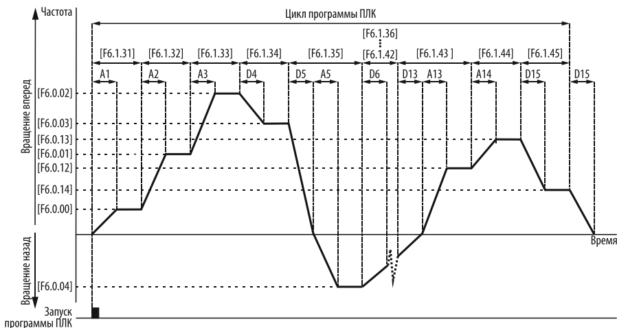
Рисунок 150 – один цикл программы ПЛК с остановкой по завершении цикла.
