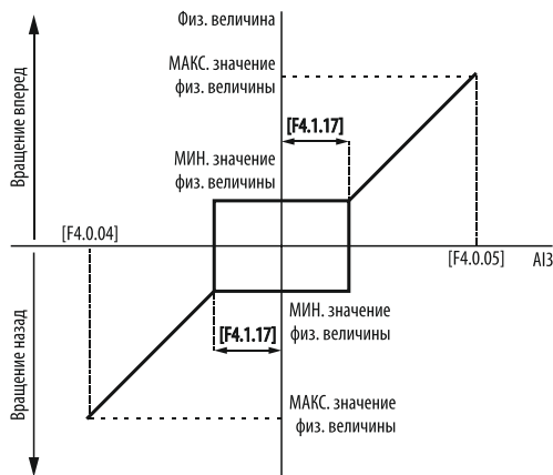
Рисунок 114 – минимальное и максимальное значение напряжения на аналоговом входе AI3 в биполярном режиме.
