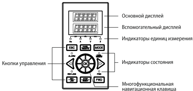
Рисунок 51 – внешний вид панели управления AFD-XPNL.22.
