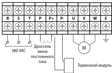
Рисунок 30 - клеммы силового терминала (модификации: AFD-E450.43, AFD-E550.43)
