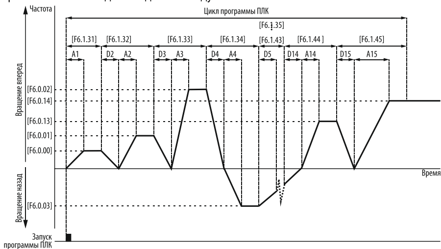
Рисунок 155 – один цикл с остановкой между шагами и работой на частоте последнего шага по окончании цикла.
