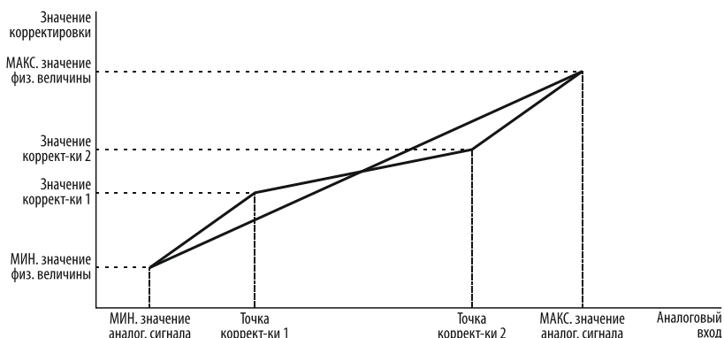
Рисунок 116 – корректировка кривой аналоговых входов AI1 , AI2 , AI3 .
