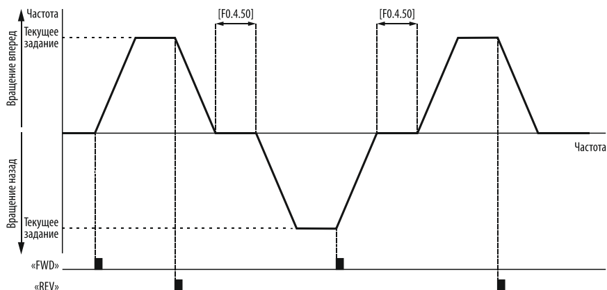
Рисунок 82 – задержка времени между прямым и реверсивным направлением вращения вала электродвигателя.
