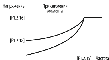
Рисунок 89 – усиление момента при работе ПЧ в U/f режиме.
