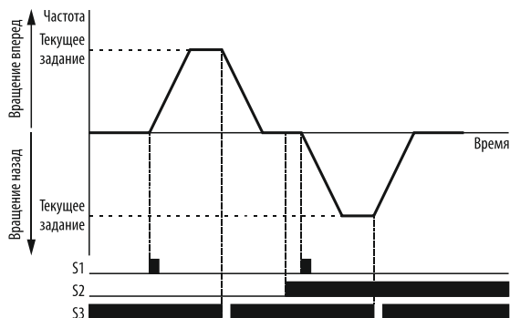
Рисунок 72 – трёхпроводной режим управления №2.
