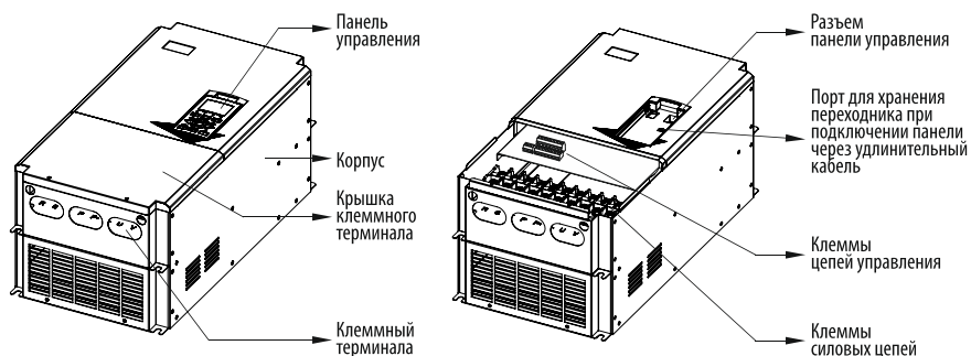
Рисунок 5 – тип корпуса 3, габариты 8, 9, 10, 11, 12 (модели AFD-E370.43...AFD-E2200.43)
