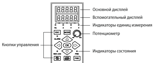
Рисунок 171 - внешний вид панели управления AFD-XPNL.12
