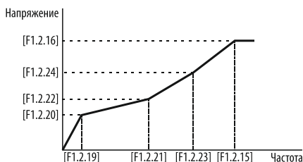
Рисунок 90 – пользовательская настройка U/f кривой.
