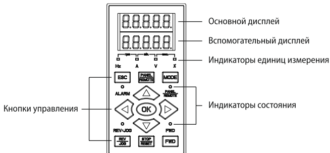
Рисунок 50 – внешний вид панели управления AFD-XPNL.11
