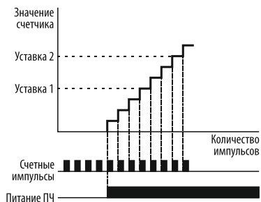
Рисунок 137 – запуск счётчика при подаче питания ПЧ.
