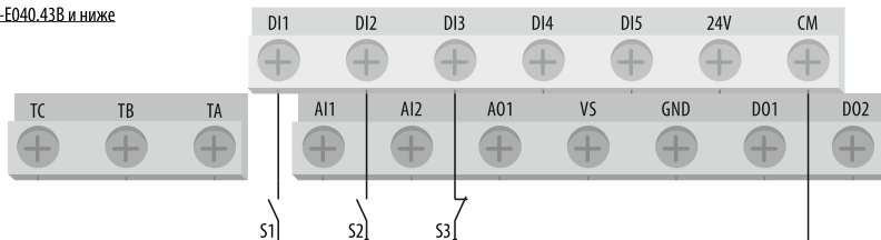
Рисунок 72 – трёхпроводной режим управления №2.
