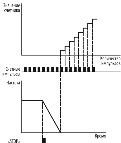
Рисунок 140 – запуск счётчика при остановке электродвигателя.
