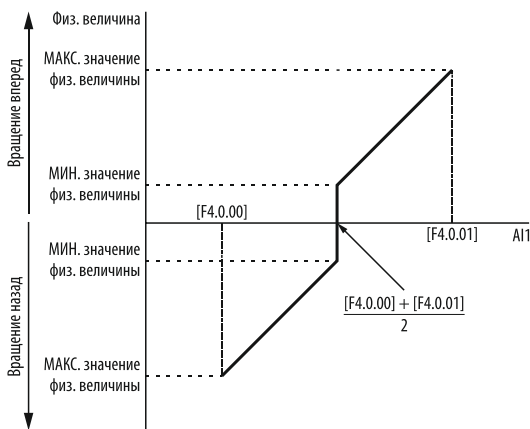
Рисунок 111 – минимальное и максимальное значение напряжения на аналоговом входе AI1 в биполярном режиме.
