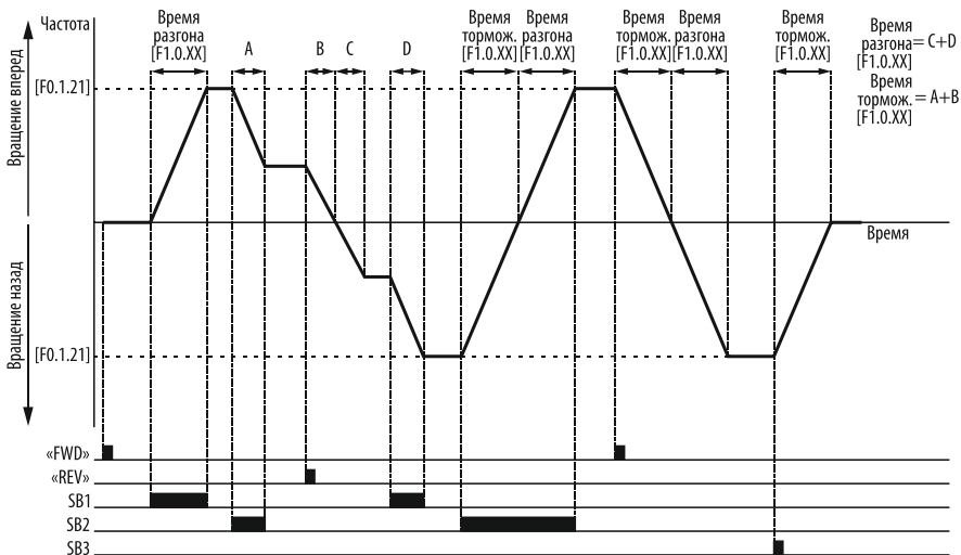
Рисунок 64 – двустороннее задание частоты с дискретных входов с возможностью управления направлением вращения.
