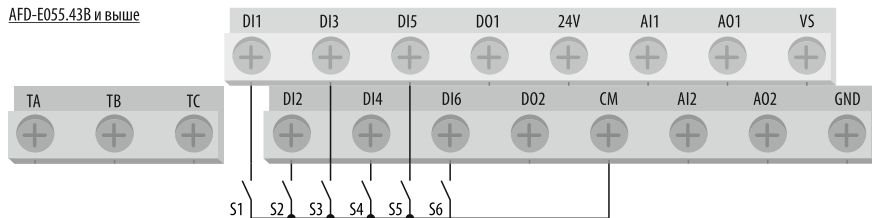
Рисунок 37 – схема подключения сигнала типа «сухой контакт» к дискретным входам (питание от внутреннего источника питания 24 В)
