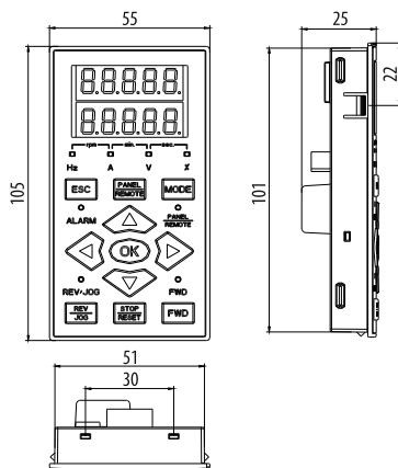
Рисунок 17 – габаритные размеры панели управления AFD-XPNL.11
