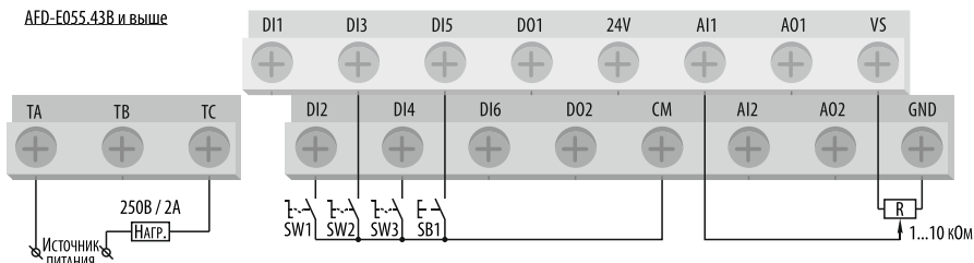
Рисунок 59 – схема подключения цепей управления при [F0.0.00] = «6».
