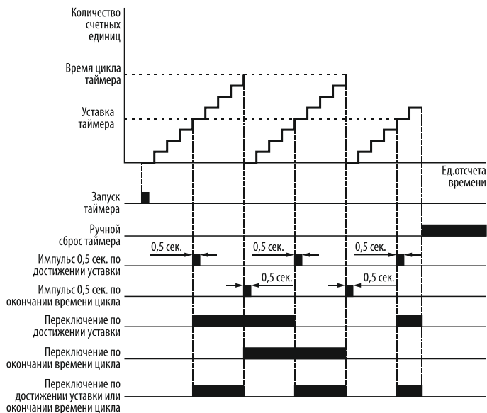
Рисунок 133 – функции выходов таймеров при циклическом режиме работы с ручным сбросом текущего значения таймера.
