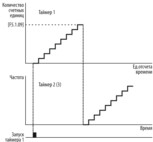
Рисунок 127 – запуск таймера 2, 3 по окончании времени цикла таймера 1.
