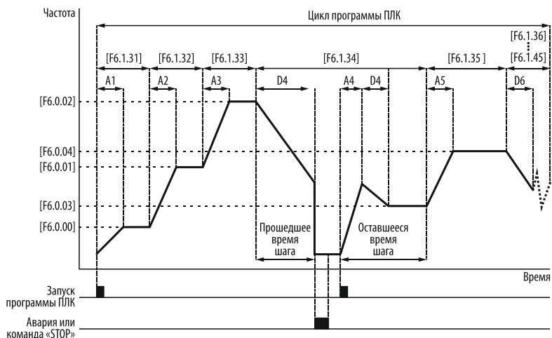
Рисунок 156 – запуск программы ПЛК с места прерывания программы.
