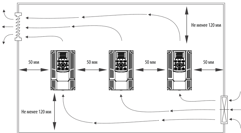
Рисунок 12 – Установка нескольких преобразователей частоты в одном шкафу.
