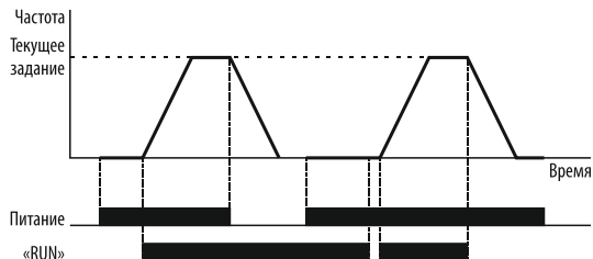
Рисунок 75 – автоматический запуск электродвигателя после включения питания «Запрещён».
