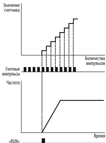
Рисунок 139 – запуск счётчика при запуске электродвигателя.
