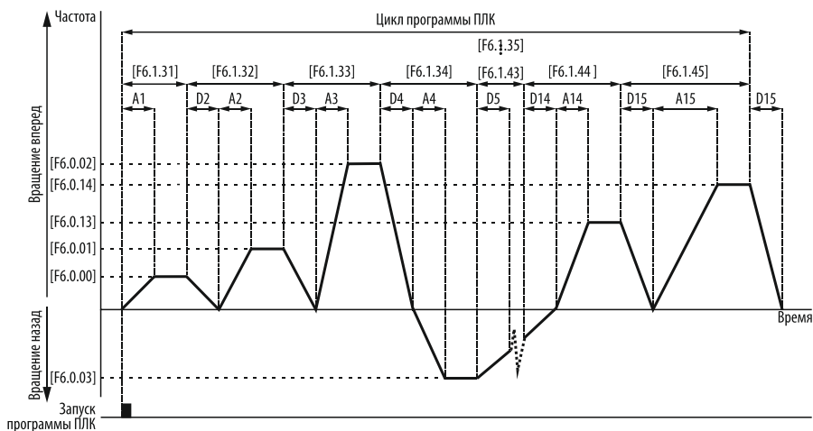
Рисунок 151 – один цикл с остановкой между шагами и остановкой по завершении цикла.
