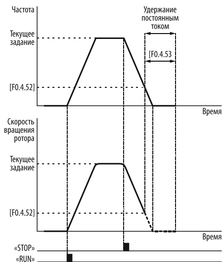
Рисунок 86 – обнаружение нулевой скорости при [F0.4.53] \neq «0» .
