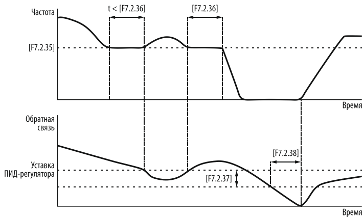
Рисунок 165 – работа ПЧ при активной функции «Сон».
