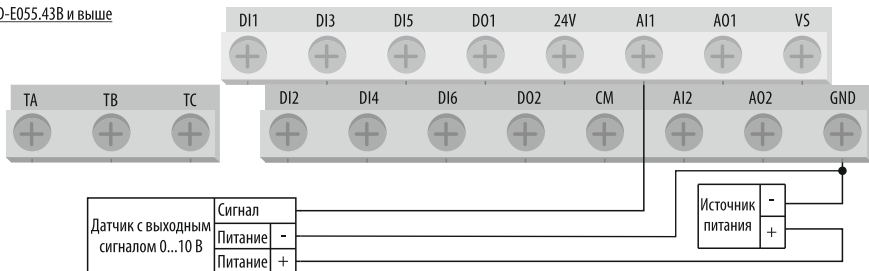
Рисунок 44 – схема подключения датчика с аналоговым выходным сигналом 0...10 В (питание от внешнего источника питания 24 В).
