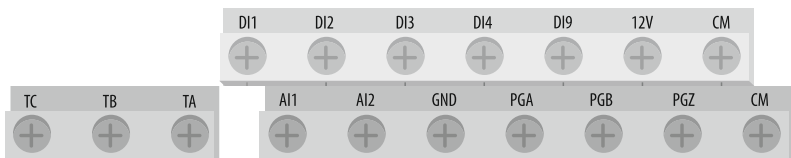
Рисунок 175 –клеммы карты расширения AFD-XPLT.A103
