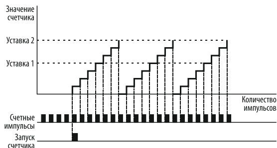
Рисунок 143 – сброс текущего значения счетчика по достижении уставки 2.
