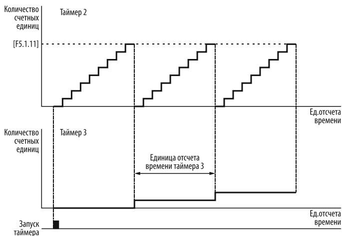
Рисунок 122 – единицы измерения таймеров 3 в завершённых циклах таймера 2.
