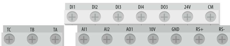
Рисунок 174 – клеммы карты расширения AFD-XPLT.A102
