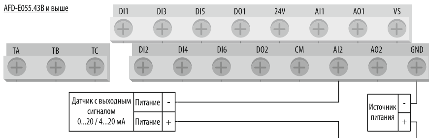
Рисунок 42 – схема подключения датчика с аналоговым выходным сигналом 0...20 / 4...20 мА (питание от внешнего источника питания 24 В).
