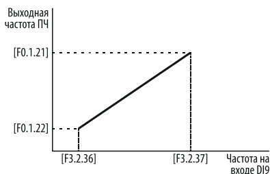
Рисунок 106 – масштабирование входного высокочастотного дискретного сигнала на высокоскоростном входе DI9 при [F0.2.25] = «14».
