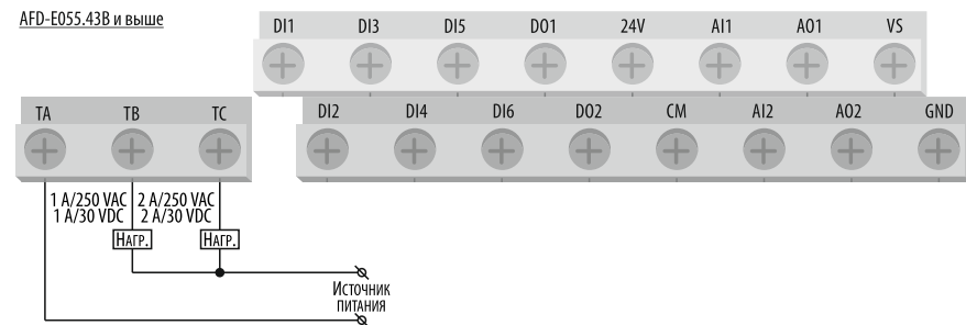
Рисунок 46 – схема подключения нагрузки к релейному выходу (питание от внешнего источника питания постоянного или переменного тока).
