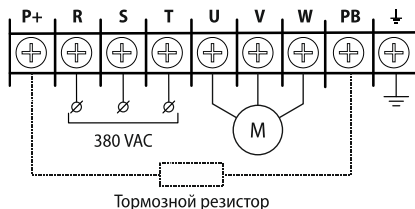
Рисунок 24 – клеммы силового терминала (модификации: AFD-E055.43B)
