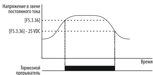
Рисунок 148 – диапазон напряжения в звене постоянного тока для включения / отключения тормозного прерывателя.
