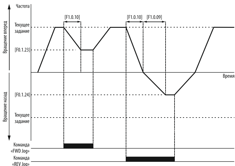
Рисунок 61 – работа ПЧ в режиме Jog.
