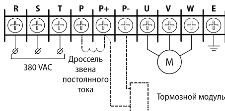
Рисунок 31 - клеммы силового терминала (модификации: AFD-E750.43, AFD-E900.43, AFD-E1100.43, AFD-E1320.43, AFD-E1600.43, AFD-E1850.43, AFD-E2000.43, AFD-E2200.43)
