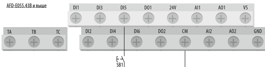
Рисунок 54 – схема подключения цепей управления при [F0.0.00] = «2» .
