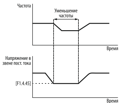
Рисунок 95 – Компенсация понижения напряжения в звене постоянного тока.
