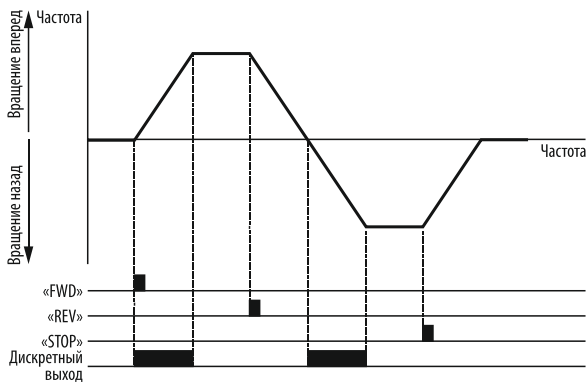
Рисунок 101– включение дискретного выхода на время разгона.
