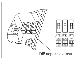
Рисунок 36 – DIP переключатели ПЧ AFD-E055.43В и выше.
