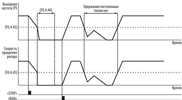
Рисунок 80 – удержание постоянным током при команде «STOP».
