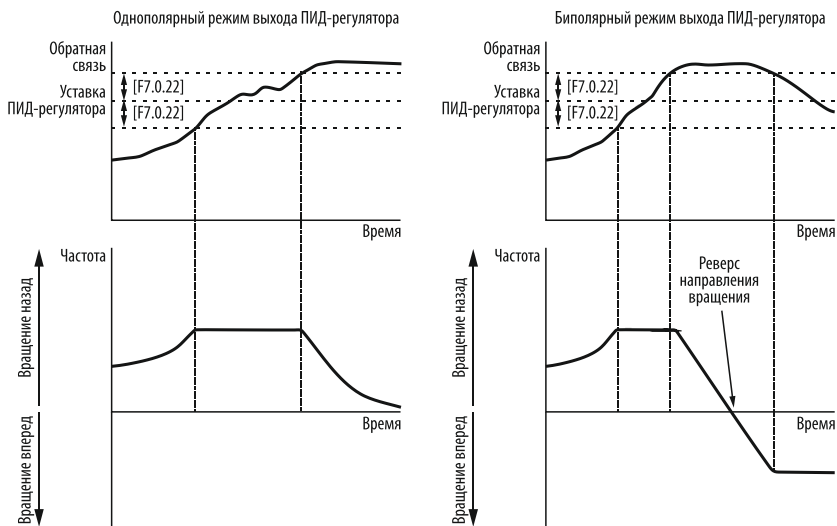
Рисунок 162 – работа встроенного ПИД-регулятора в однополярном и биполярном режимах.
