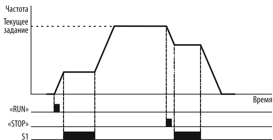
Рисунок 97 – задержка разгона и торможения.
