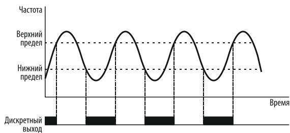
Рисунок 103 – включение дискретного выхода при достижении параметром мониторинга значения ниже нижнего предела.
