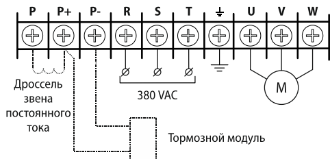
Рисунок 28 - клеммы силового терминала (модификации: AFD-E300.43)
