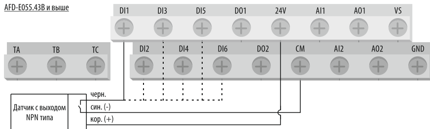
Рисунок 38 – схема подключения датчиков с выходом NPN типа к дискретным входам (питание от внутреннего источника питания 24 В).
