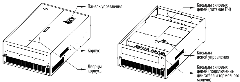
Рисунок 6 - тип корпуса 4, габарит 13 (модели AFD-E2500.43...AFD-E3150.43)
