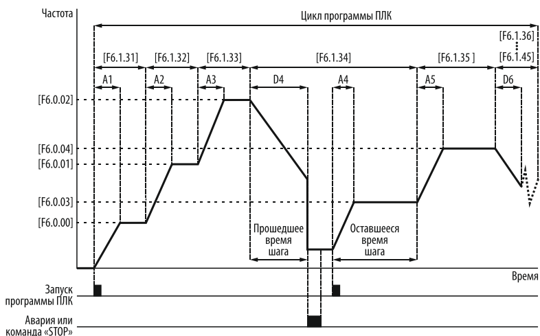
Рисунок 157 – запуск программы ПЛК с частоты шага прерывания программы.
