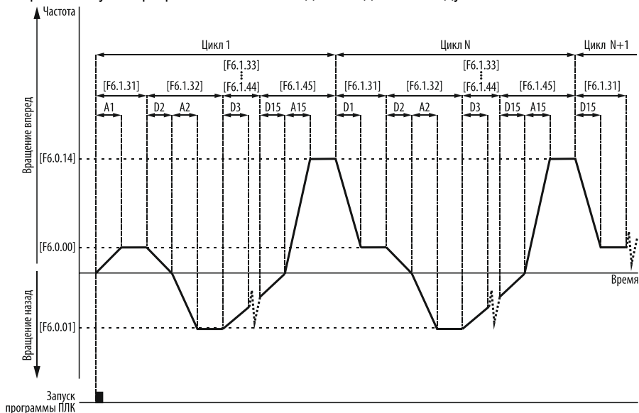
Рисунок 152 – циклическое выполнение программы.
