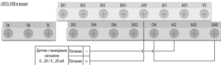
Рисунок 41 – Схема подключения датчика с аналоговым выходным сигналом 0...20 / 4...20 мА (питание от внутреннего источника питания 24 В).
