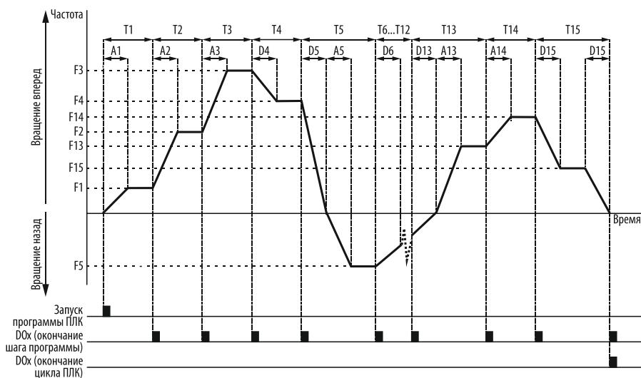
Рисунок 149 – основные параметры программы встроенного ПЛК.
