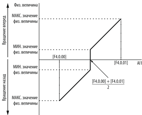
Рисунок 65 – двусторонне задание частоты при помощи аналогового входа AI1.
