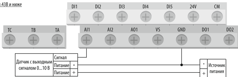
Рисунок 43 – схема подключения датчика с аналоговым выходным сигналом 0...10 В (питание от внутреннего источника питания 24 В).
