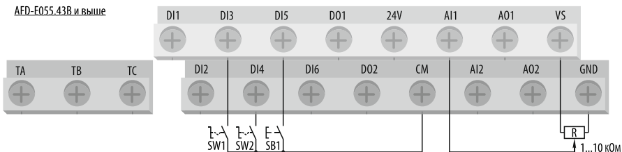
Рисунок 57 – схема подключения цепей управления при [F0.0.00] = «4» для AFD-E055.43B и выше.
