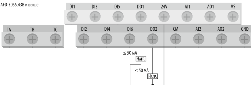
Рисунок 47 – схема подключения нагрузки к транзисторному выходу (питание от внутреннего источника питания 24 В).
