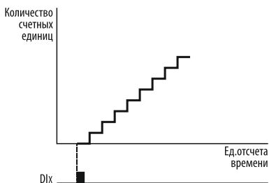
Рисунок 123 – запуск таймера по сигналу на дискретном входе.
