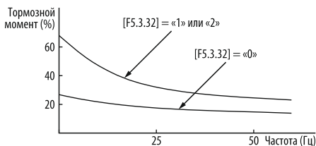
Рисунок 147 – изменение тормозного момента после применения торможения магнитным потоком.
