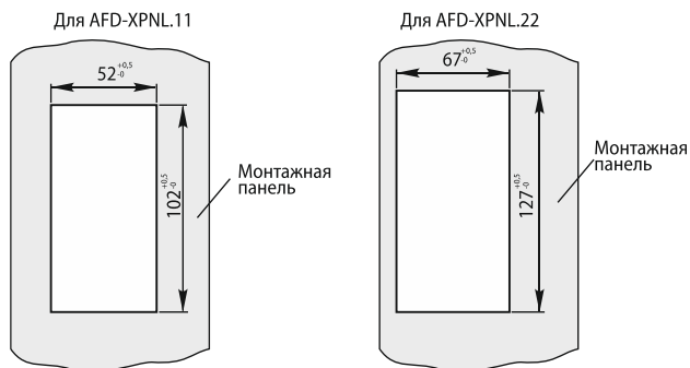
Рисунок 19 – размеры монтажного отверстия для выносного монтажа панелей управления AFD-XPNL 11 (слева) и AFD-XPNL 22 (справа)
