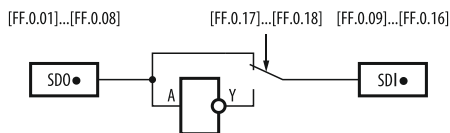
Рисунок 170 – функциональная схема работы виртуальных входов / выходов.
