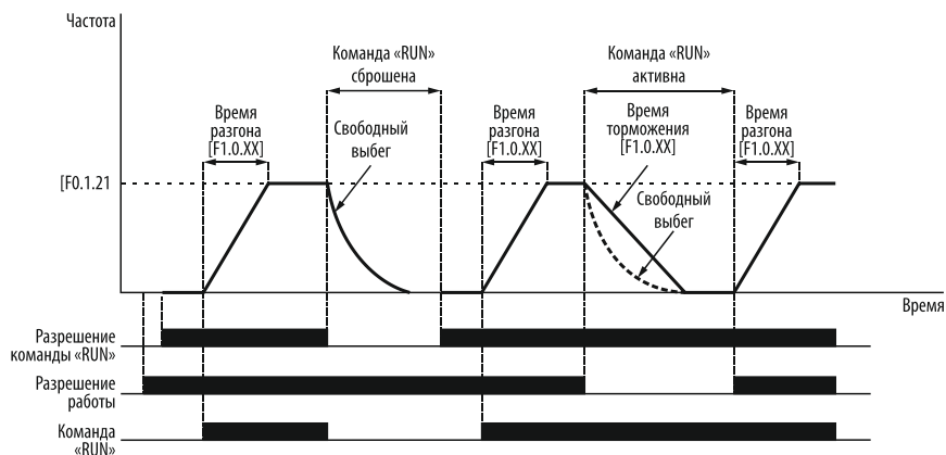
Рисунок 76 – разрешение команды «RUN» и разрешение работы.
