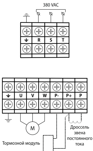
Рисунок 32 - клеммы силового терминала (модификации: AFD-E2500.43, AFD-E3150.43)
