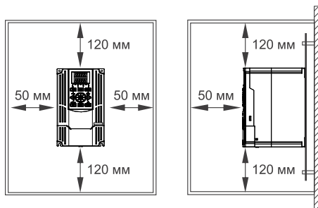
Рисунок 9 – минимально допустимые расстояния от ПЧ до окружающих предметов.
