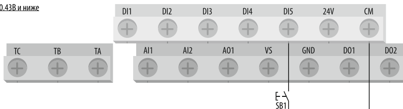
Рисунок 52 – схема подключения цепей управления при [F0.0.00] = «1» для AFD-E040.43B и ниже.
