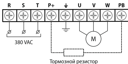
Рисунок 23 – клеммы силового терминала (модификации: AFD-E022.43B, AFD-E040.43B)
