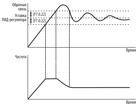
Рисунок 163 – допустимая статическая ошибка.
