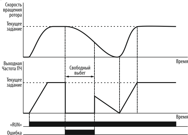
Рисунок 77 – режим запуска с поиском скорости.
