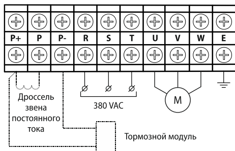
Рисунок 29 - клеммы силового терминала (модификации: AFD-E370.43)
