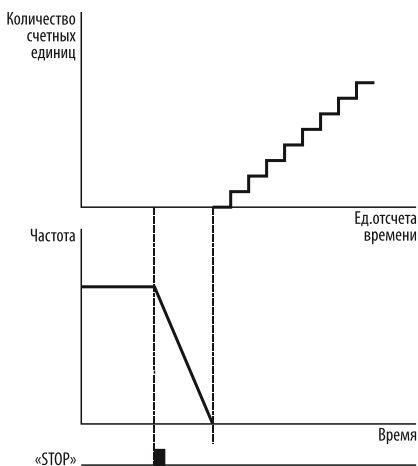
Рисунок 125– запуск таймера при остановке электродвигателя.
