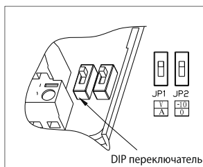
Рисунок 35 – DIP переключатели ПЧ AFD-E040.43В и ниже.
