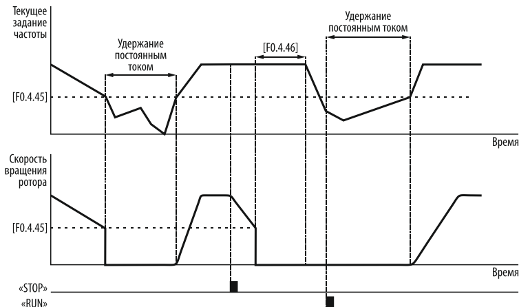
Рисунок 81 – удержание постоянным током при достижении заданной частоты.
