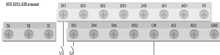
Рисунок 70 – подключение внешних управляющих сигналов при двухпроводном режиме управления №1 и №2.
