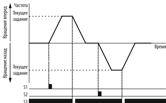
Рисунок 71 – трёхпроводной режим управления №1.
