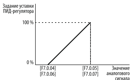
Рисунок 160 – масштабирование задания ПИД-регулятора относительно аналогового сигнала.
