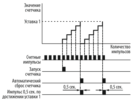
Рисунок 145– автоматический сброс текущего значения счетчика по достижении уставки 1.
