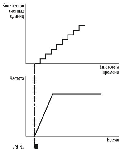
Рисунок 124 – запуск таймера при запуске электродвигателя.
