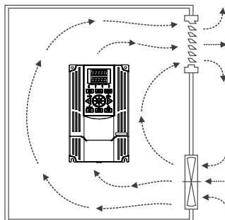
Рисунок 11 – расположение элементов системы дополнительной вентиляции.
