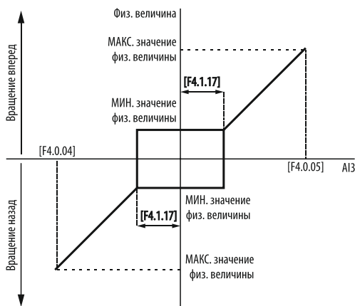
Рисунок 115 – гистерезис аналогового сигнала на входе AI3 в биполярном режиме.
