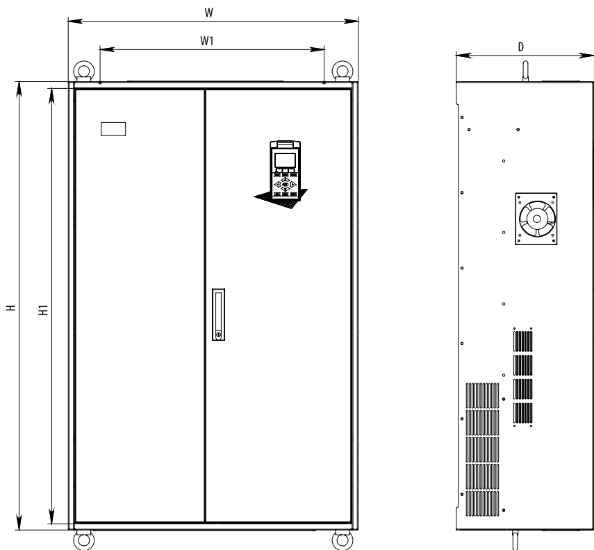
Рисунок 16 - габаритные размеры AFD-E2500.43 и выше (тип корпуса 4, габарит 13)
