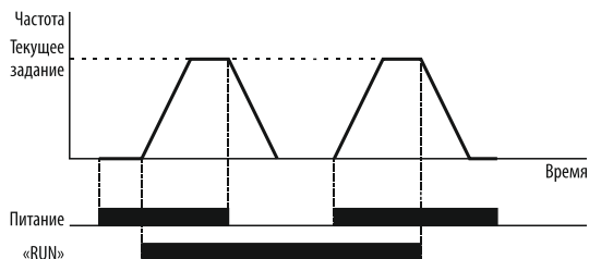
Рисунок 74 – автоматический запуск электродвигателя после включения питания «Разрешён».
