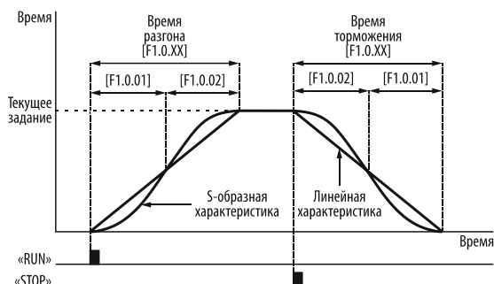
Рисунок 87 – характеристики разгона и торможения.
