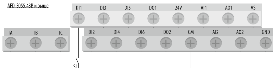
Рисунок 99 – пример схемы подключения внешних сигналов для при использовании функции «21» для ПЧ AFD-E055.43B и выше.
