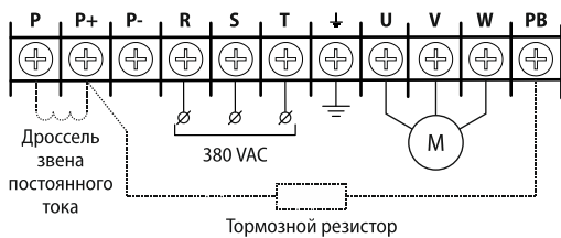
Рисунок 26 - клеммы силового терминала (модификации: AFD-E150.43B, AFD-E185.43B)
