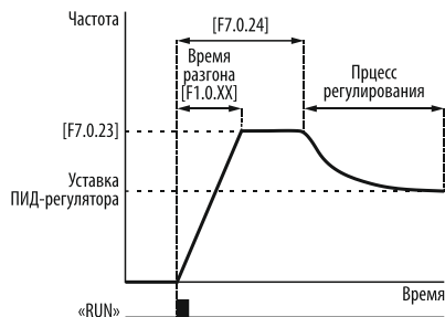
Рисунок 164 – Работа ПИД-регулятора на предустановленной частоте.
