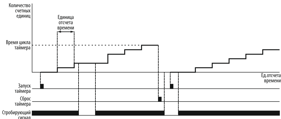
Рисунок 130– применение стробящего сигнала для таймеров 1, 2, 3.
