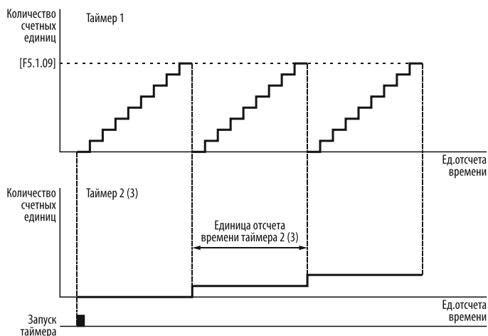
Рисунок 121 – единицы измерения таймеров 2 и 3 в завершённых циклах таймера 1.
