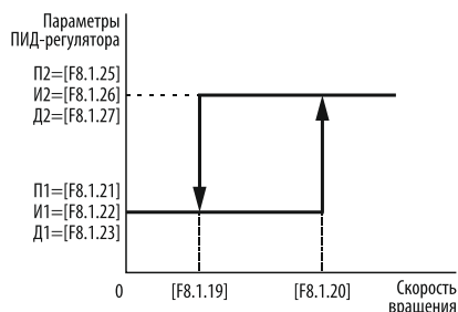
Рисунок 168 – переключение между ПИД1 и ПИД2 по гистерезису.
