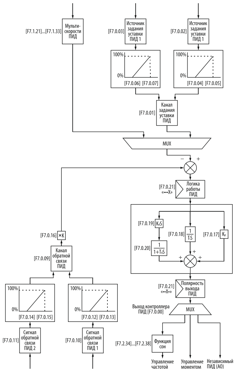
Рисунок 159 – блок-схема встроенного ПИД-регулятора.
