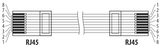
Рисунок 49 – схема кабеля для подключения панели управления к ПЧ при выносном монтаже. (Тип кабеля: экранированный сетевой кабель Cat.5e, тип разъёма: RJ-45, разводка: TIA / EIA-T568B).
