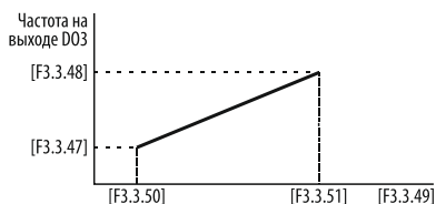
Рисунок 109 – масштабирование параметра мониторинга относительно диапазона выходной частоты на выходе DO3 .
