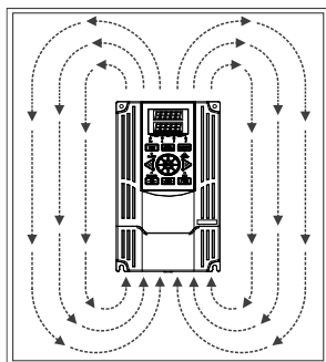
Рисунок 10 – Циркуляция воздуха в герметичном шкафу без системы дополнительного охлаждения.
