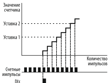
Рисунок 138 – запуск счётчика по сигналу на дискретном входе.
