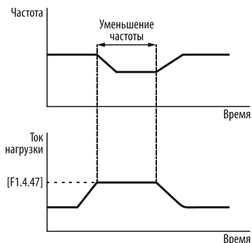
Рисунок 96 – Компенсация повышения тока нагрузки.
