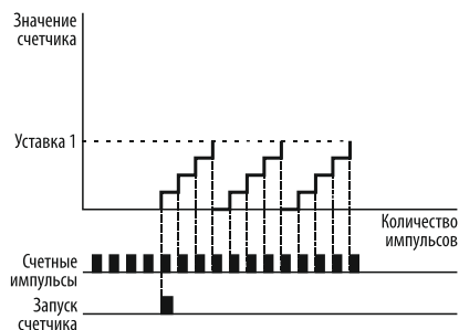
Рисунок 142 – сброс текущего значения счётчика по достижении уставки 1.
