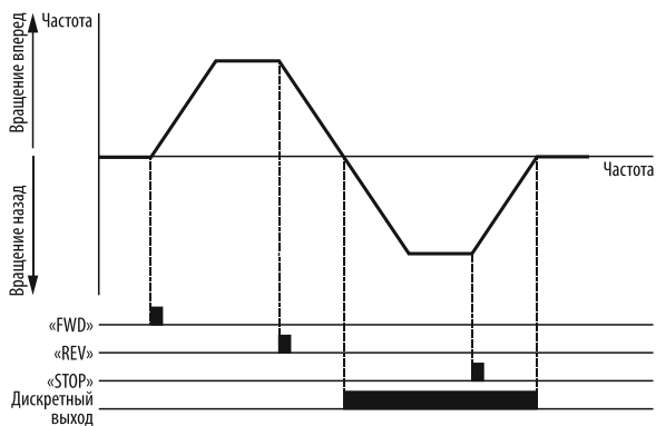
Рисунок 100 – включение дискретного выхода при включении реверса электродвигателя.
