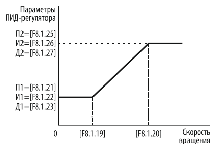
Рисунок 169 – непрерывное переключение между ПИД1 и ПИД2.
