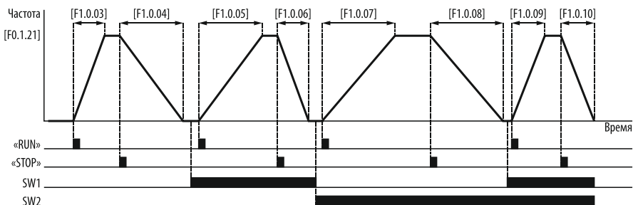
Рисунок 88 – выбор времени разгона и торможения при помощи сигналов на дискретных входах.
