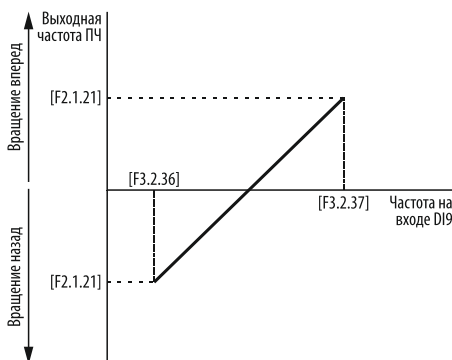
Рисунок 107 – масштабирование входного высокочастотного дискретного сигнала на высокоскоростном входе DI9 при [F0.2.25] = «15».
