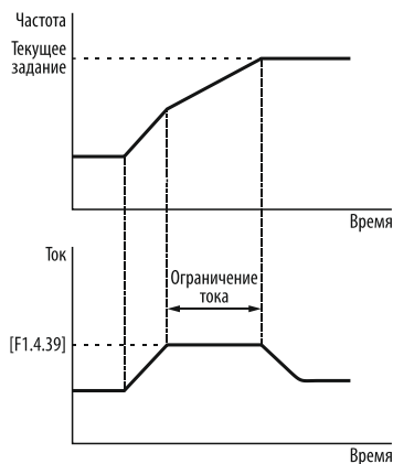
Рисунок 92– ограничение тока нагрузки при разгоне.
