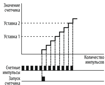
Рисунок 135 – счёт импульсов по заднему фронту импульсов.
