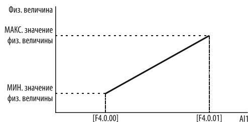
Рисунок 110 – минимальное и максимальное значение напряжения на аналоговом входе A11 .
