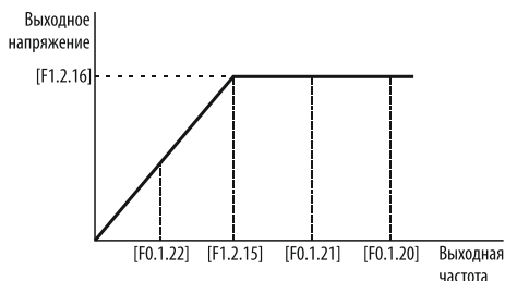
Рисунок 60 – распределение «Максимальной выходной частоты», «верхнего предела частоты» и «нижнего предела частоты» в настройках ПЧ.
