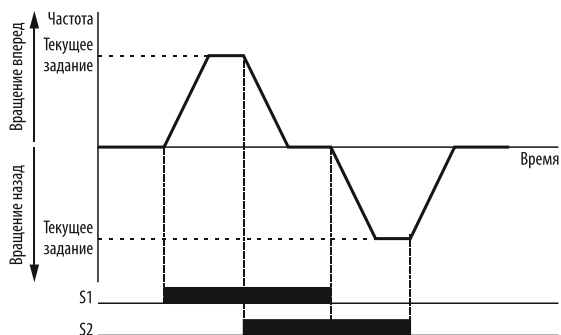
Рисунок 68 – двухпроводной режим управления №1.
