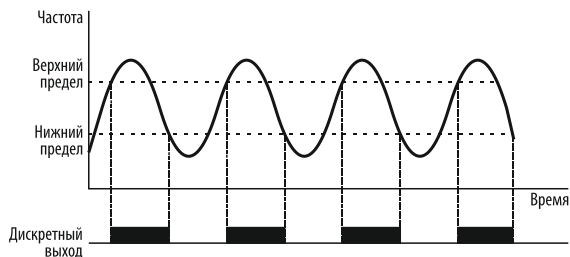
Рисунок 104 – включение дискретного выхода при достижении параметром мониторинга значения выше верхнего предела.
