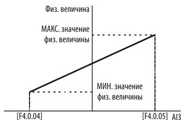
Рисунок 113 – минимальное и максимальное значение напряжения на аналоговом входе AI3 в униполярном режиме.
