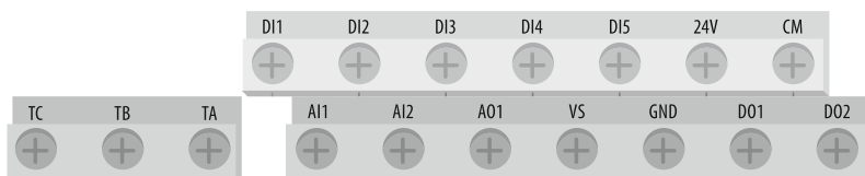
Рисунок 33 – клеммы цепей управления ПЧ AFD-E040.43B и ниже
