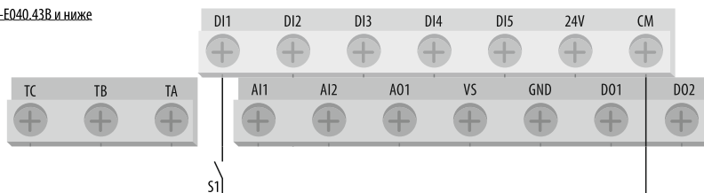
Рисунок 98 – пример схемы подключения внешних сигналов для при использовании функции «21» для ПЧ AFD-E040.43B и ниже.
