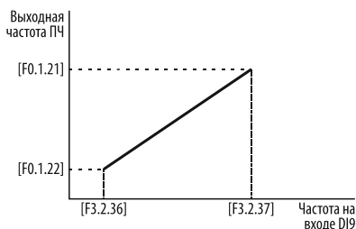
Рисунок 66 – задание частоты при помощи сигнала на высокоскоростном дискретном входе DI9.
