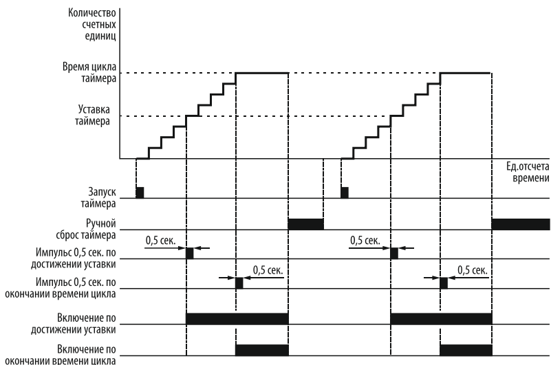
Рисунок 131 – функции выходов таймеров при одиночном цикле с ручным сбросом текущего значения таймера.
