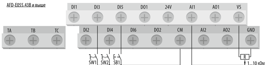
Рисунок 55 – схема подключения цепей управления при [F0.0.00] = «3» .
