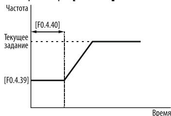
Рисунок 78 – стартовая частота и время работы на стартовой частоте.
