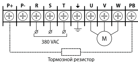
Рисунок 25 – клеммы силового терминала (модификации: AFD-E075.43B, AFD-E090.43B, AFD-E110.43B)
