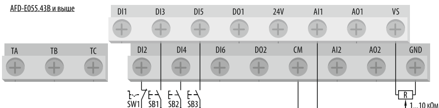
Рисунок 58 – Схема подключения цепей управления при [F0.0.00] = «5»
