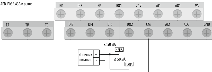
Рисунок 48 – схема подключения нагрузки к транзисторному выходу (питание от внешнего источника питания 24 В).
