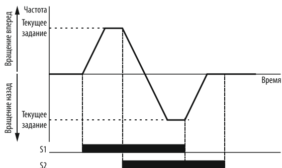
Рисунок 69 – двухпроводной режим управления №2.
