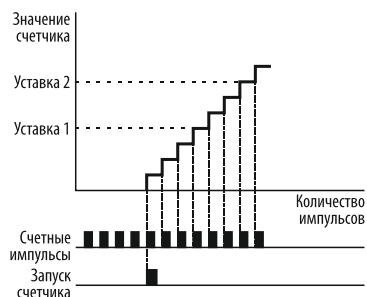
Рисунок 134 – счет импульсов по переднему фронту импульсов.
