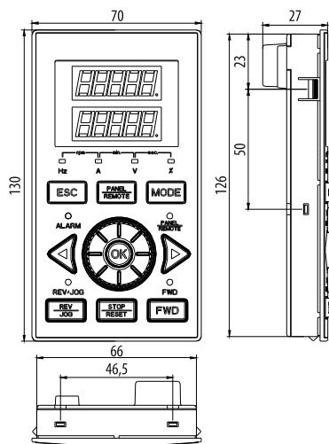
Рисунок 18 – габаритные размеры панели управления AFD-XPNL.22
