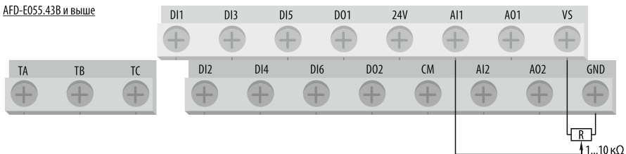
Рисунок 40 – схема подключения внешнего потенциометра (1...10 кОм).
