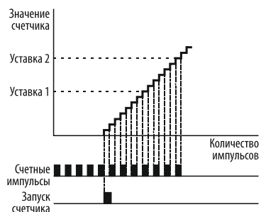
Рисунок 136 – счет импульсов по переднему и заднему фронту импульсов.
