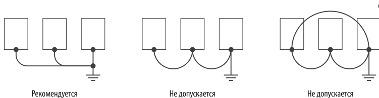
Рисунок 20 – рекомендуемая схема заземления нескольких ПЧ
