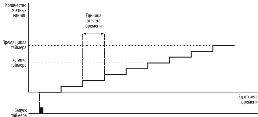
Рисунок 120– базовые параметры таймера
