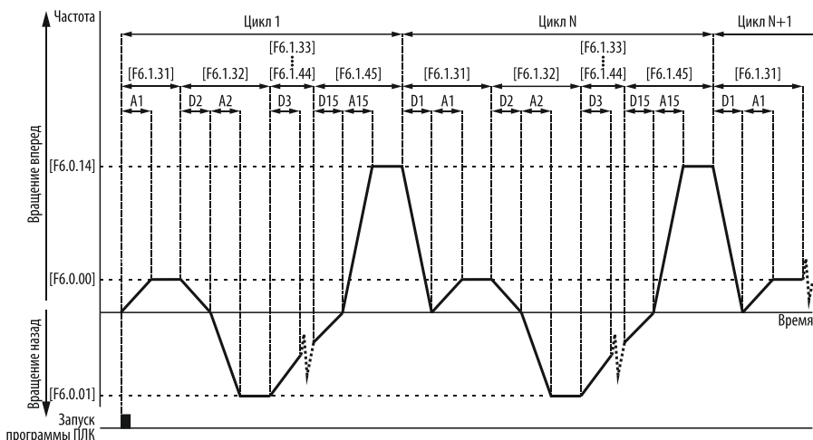
Рисунок 153— циклическое выполнение программы с остановкой между шагами.
