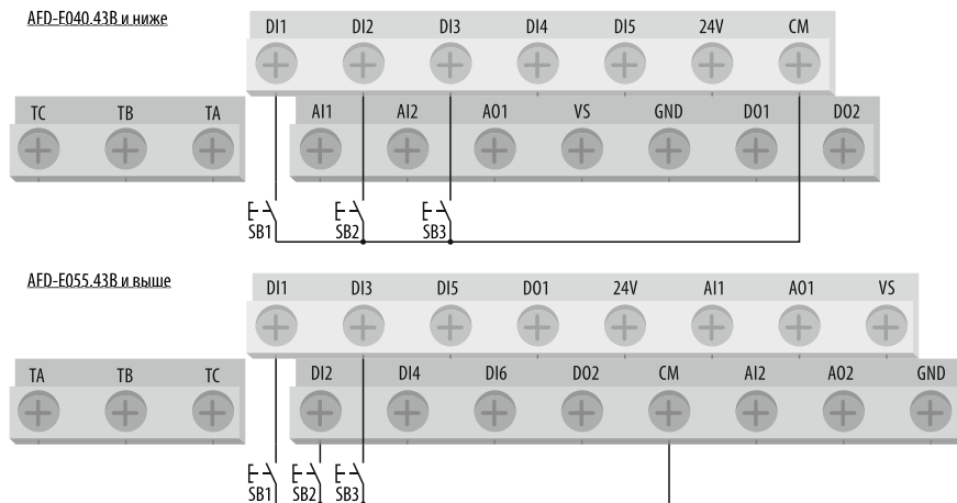
Рисунок 62 – схема подключения внешних сигналов при задании частоты с дискретных входов.
