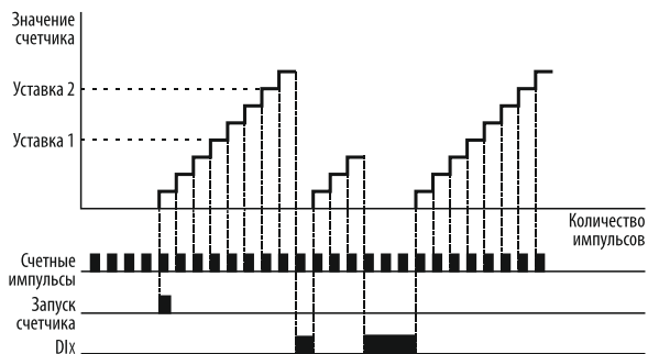
Рисунок 141 – сброс текущего значения счетчика по сигналу на дискретном входе.
