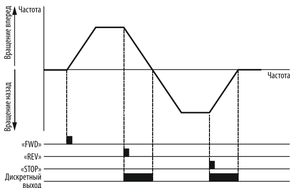
Рисунок 102 – включение дискретного выхода на время торможения.
