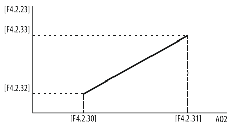
Рисунок 118 – масштабирование значения параметра мониторинга относительно диапазона выходного сигнала на выходе AO2.
