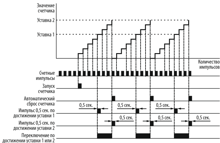
Рисунок 146– автоматический сброс текущего значения счётчика по достижении уставки 2.
