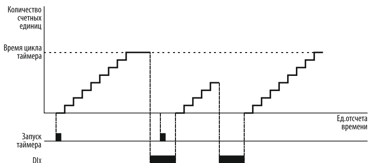
Рисунок 129 – сброс текущего значения таймера по команде на дискретном входе.
