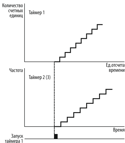
Рисунок 126 – синхронный запуск таймера 2, 3 с таймером 1.
