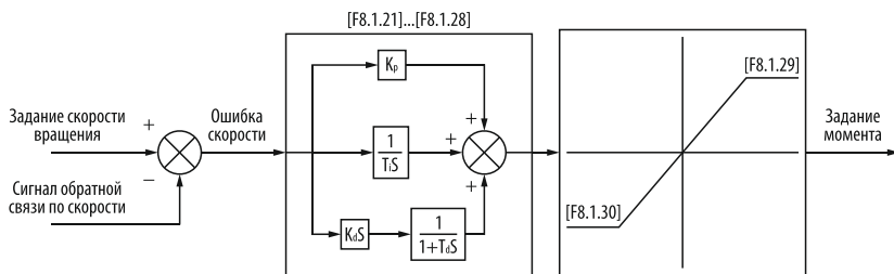
Рисунок 166 – блок-схема регулятора скорости.
