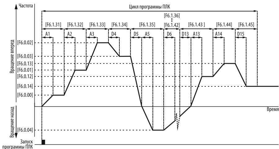
Рисунок 154 – один цикл с работой на частоте последнего шага по окончании цикла.
