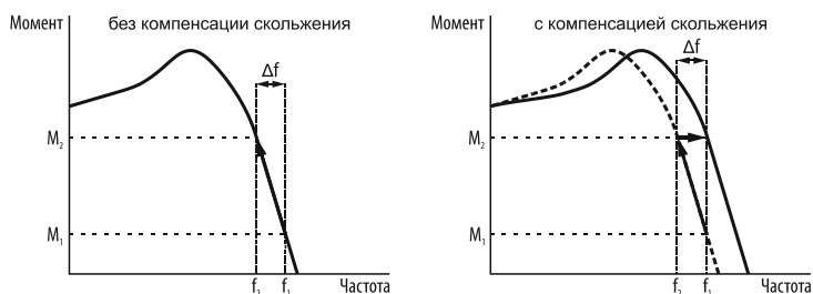
Рисунок 91 – компенсация скольжения ротора.
