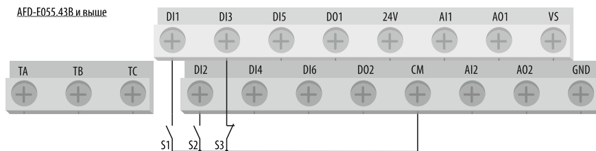
Рисунок 73 – подключение внешних управляющих сигналов при трёхпроводном режиме управления №1 и №2.
