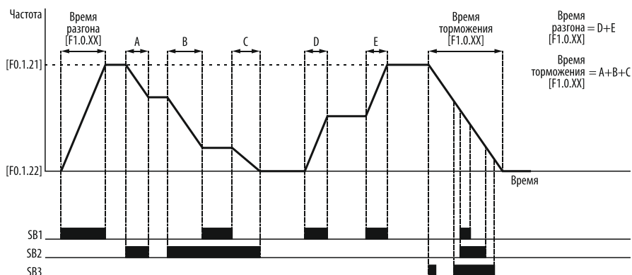
Рисунок 63 – управление выходной частотой при помощи сигналов на дискретных входах.
