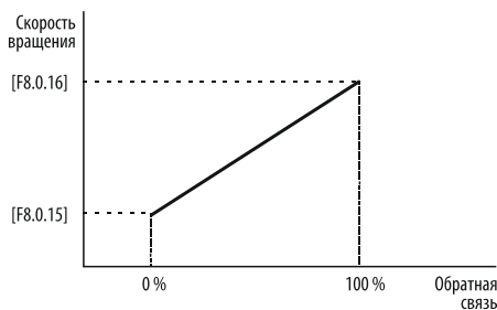
Рисунок 167 – соответствие скорости вращения электродвигателя значению сигнала обратной связи.
