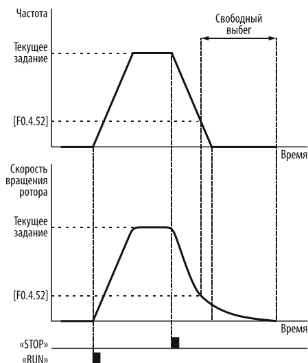
Рисунок 85 – обнаружение нулевой скорости при [F0.4.53] = «0».
