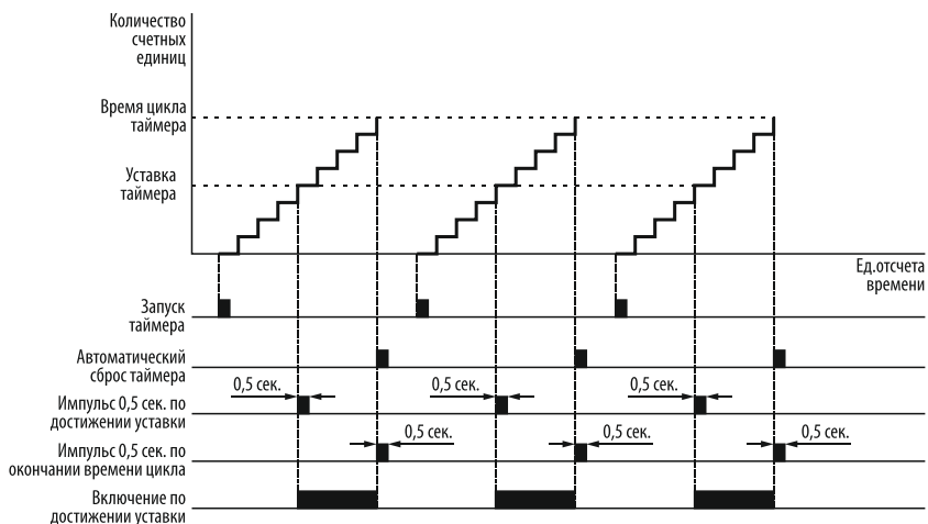
Рисунок 132 – функции выходов таймеров при одиночном цикле с автоматическим сбросом текущего значения таймера.
