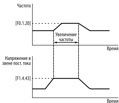
Рисунок 93 – компенсация повышения напряжения в звене постоянного тока во время работы.
