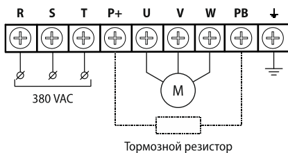
Рисунок 22 – клеммы силового терминала (модификации: AFD-E011.43B, AFD-E015.43B)
