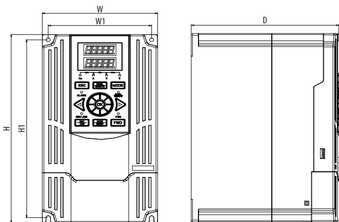
Рисунок 14 – габаритные размеры AFD-E055.43В...AFD-E300.43 (тип корпуса 2, габариты 3, 4, 5, 6, 7)
