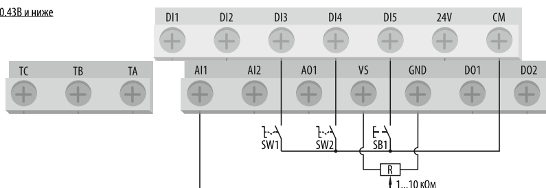
Рисунок 56 – схема подключения цепей управления при [F0.0.00] = «4» для AFD-E040.43B и ниже.
