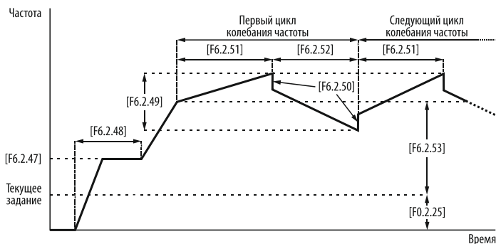
Рисунок 158 – основные параметры режима колебания частоты.
