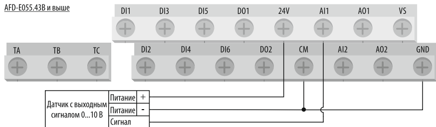
Рисунок 43 – схема подключения датчика с аналоговым выходным сигналом 0...10 В (питание от внутреннего источника питания 24 В).
