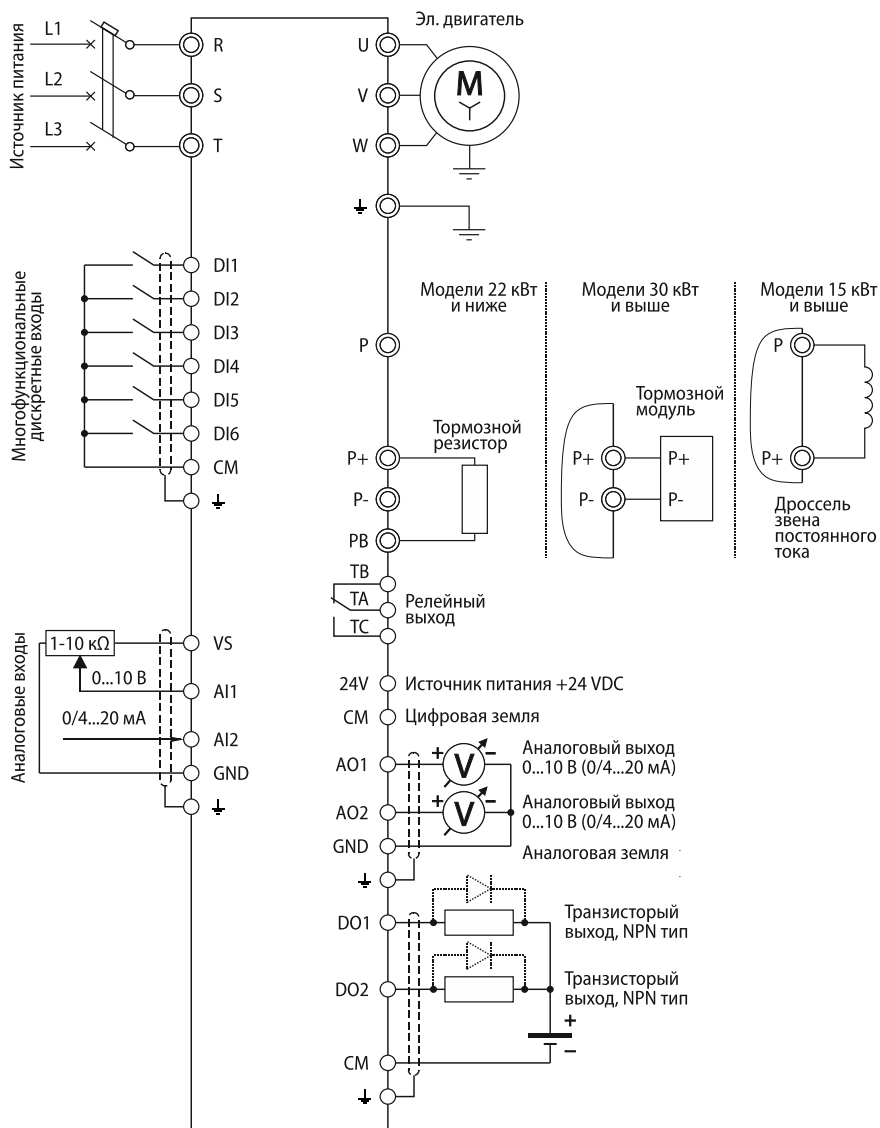
Рисунок 21 – общая схема подключения
