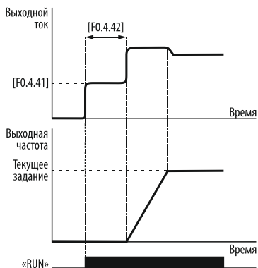
Рисунок 79 – запуск электродвигателя с предвозбуждением.
