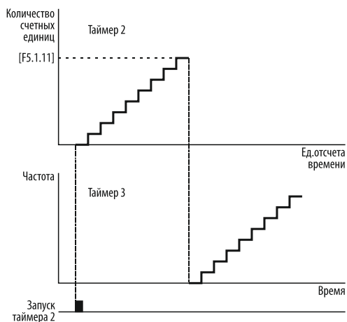
Рисунок 128 – запуск таймера 3 по окончании времени цикла таймера 2.
