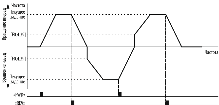
Рисунок 84 – переключение реверса при стартовой частоте.
