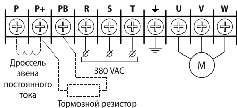
Рисунок 27 - клеммы силового терминала (модификации: AFD-E220.43B)
