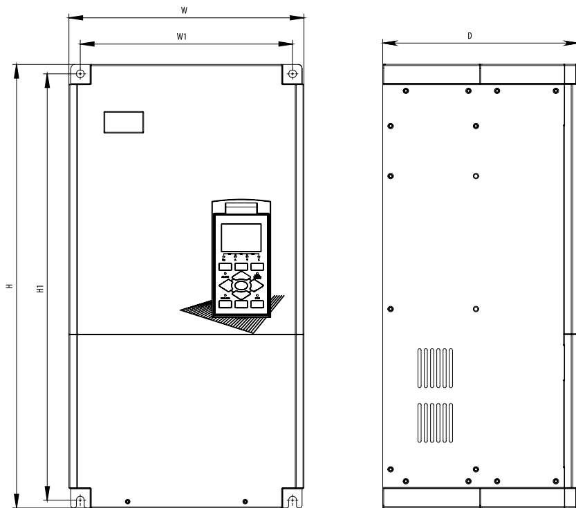
Рисунок 15 – габаритные размеры AFD-E370.43...AFD-E2200.43 (тип корпуса 3, габариты 8, 9, 10, 11, 12)
