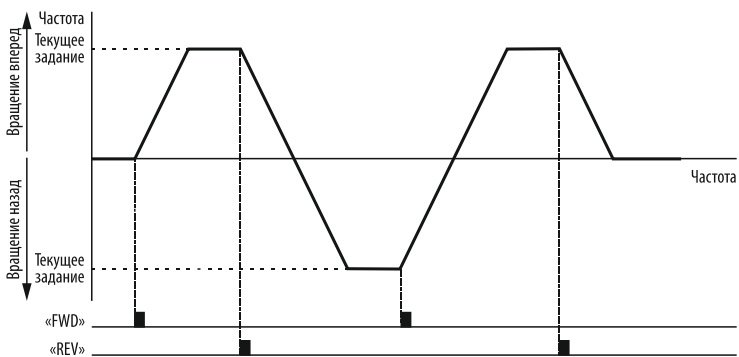
Рисунок 83 – переключение реверса при нулевой частоте
