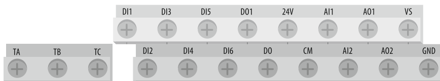
Рисунок 34 – клеммы цепей управления ПЧ AFD-E055.43B и выше
