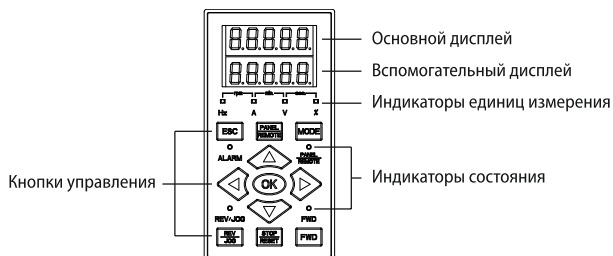
Рисунок 7 – внешний вид панели управления AFD-XPNL.11
