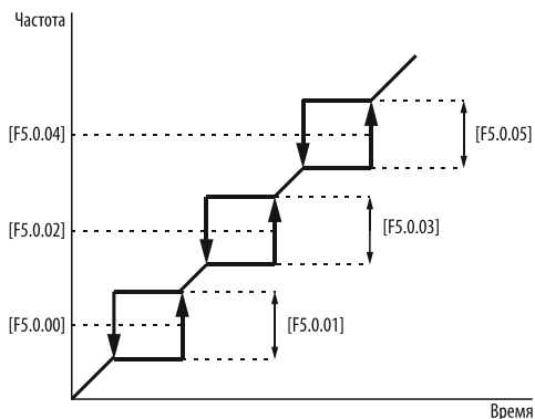
Рисунок 119 – скачкообразное изменение выходной частоты ПЧ.
