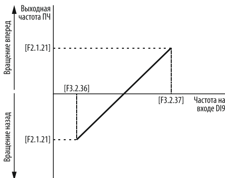
Рисунок 67 – двустороннее задание частоты при помощи сигнала на высокоскоростном дискретном входе DI9.
