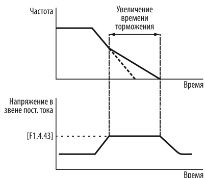
Рисунок 94 – компенсация повышения напряжения в звене постоянного тока при торможении.
