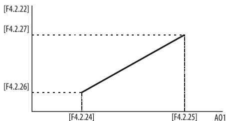
Рисунок 117 – масштабирование значения параметра мониторинга относительно диапазона выходного сигнала на выходе А01.
