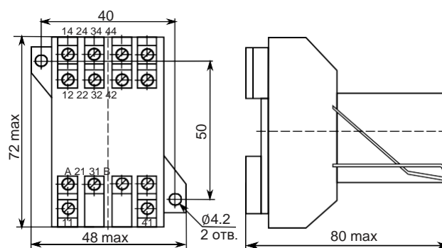
Реле с 4-мя контактами с розетками тип 3, 3А
