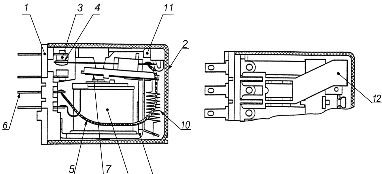
Рисунок 1. Устройство реле
