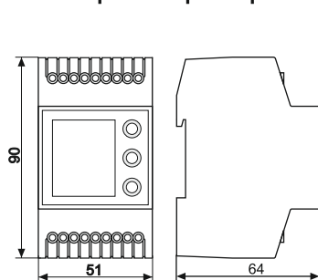
Габаритные размеры
