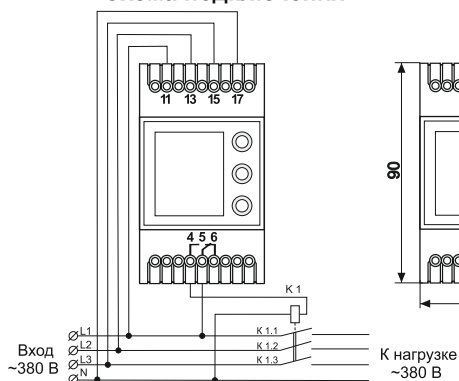
Схема подключения
